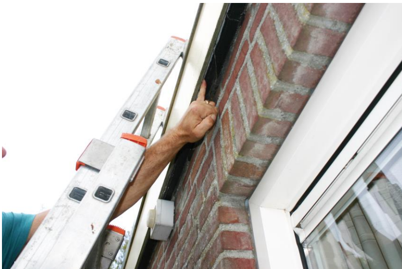
Figuur 6. Kier tussen trespa plaat en dragende lat.
