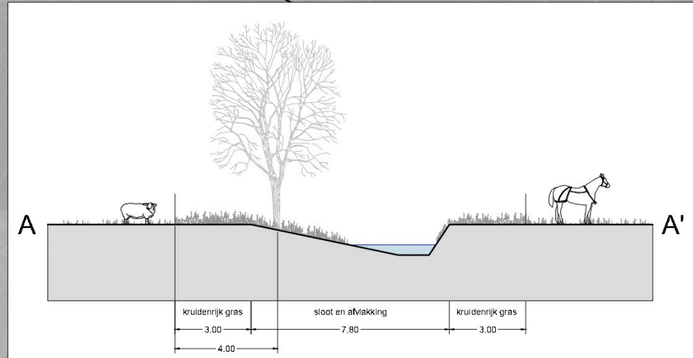
principeddoorsnede afvlakking sloot
