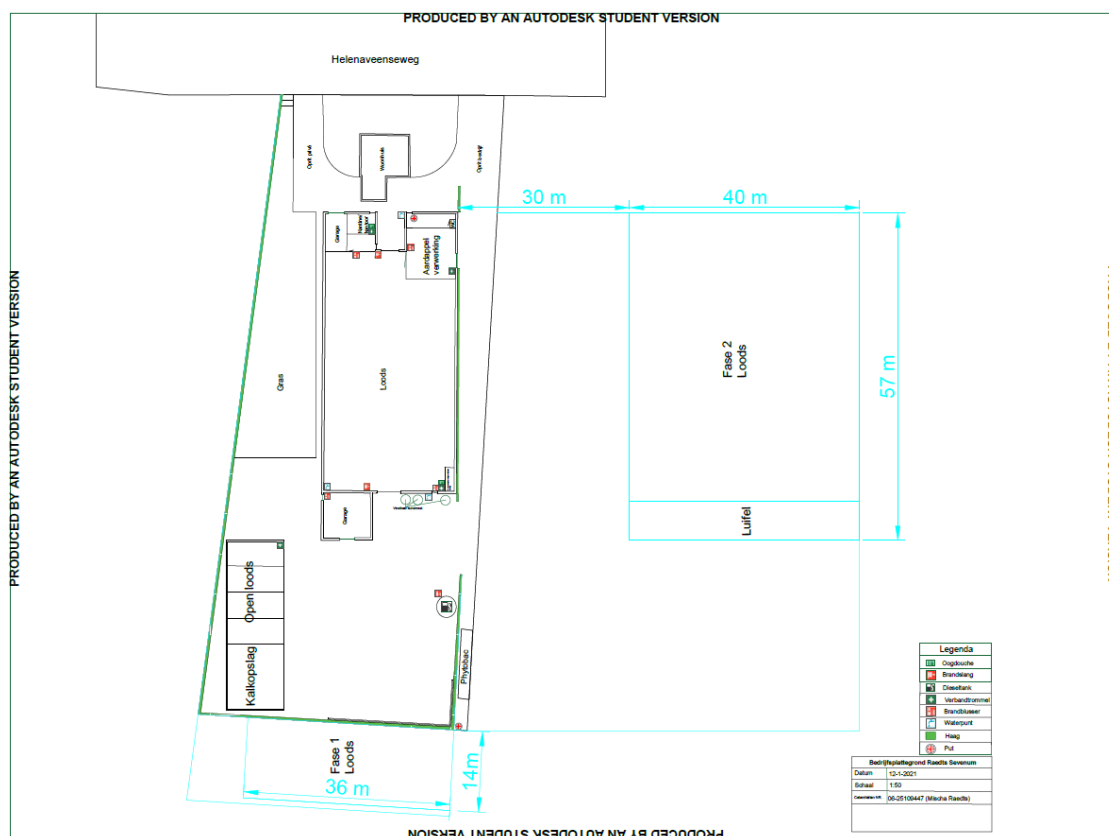
Figuur 3.1. Schets van de voorgestane situatie.
