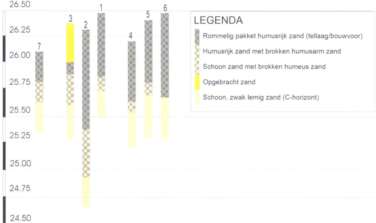
Figuur 23: Boorprofielen
