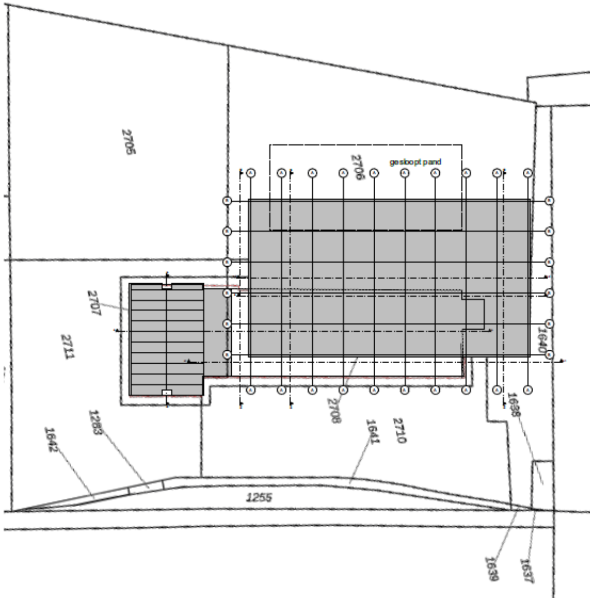
Figuur 3.1.1. Plattegrond voorgestane situatie. Bron: mc-architecten b.v./architectenbureau bna.
