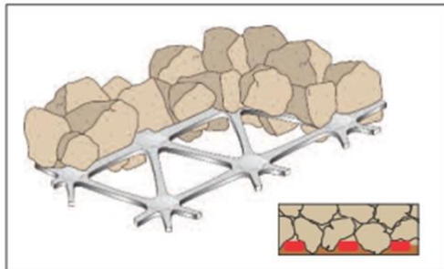
Het principe van insluiting: "interlocking"
